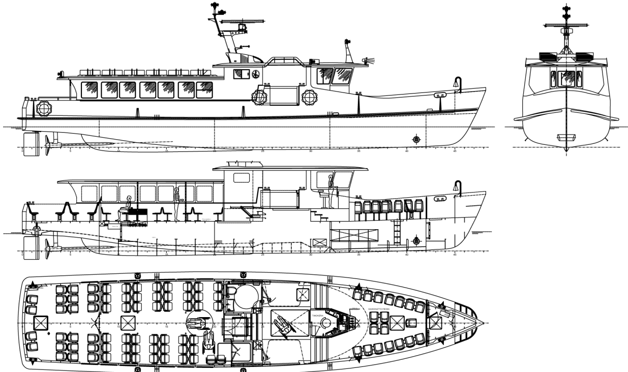
Figure 5. Passenger ferry of the Airone type. Scale 1:200. Image courtesy of Gestione Generale Navigazione Laghi.
